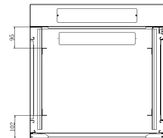
A-A Section
